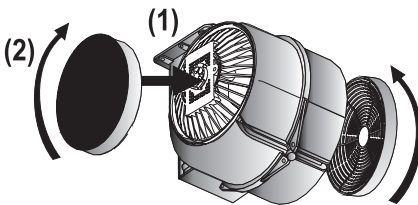
Abb.10: Einsetzen des Aktivkohlefilters AF110
