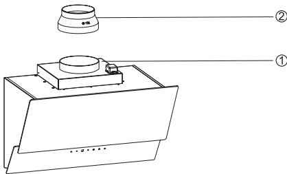
Abb. 3: Abluftstutzen-Teile
